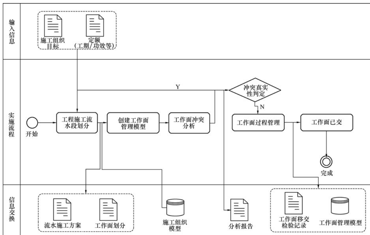
图 8.3.5 施工工作面管理 BIM 应用流程
