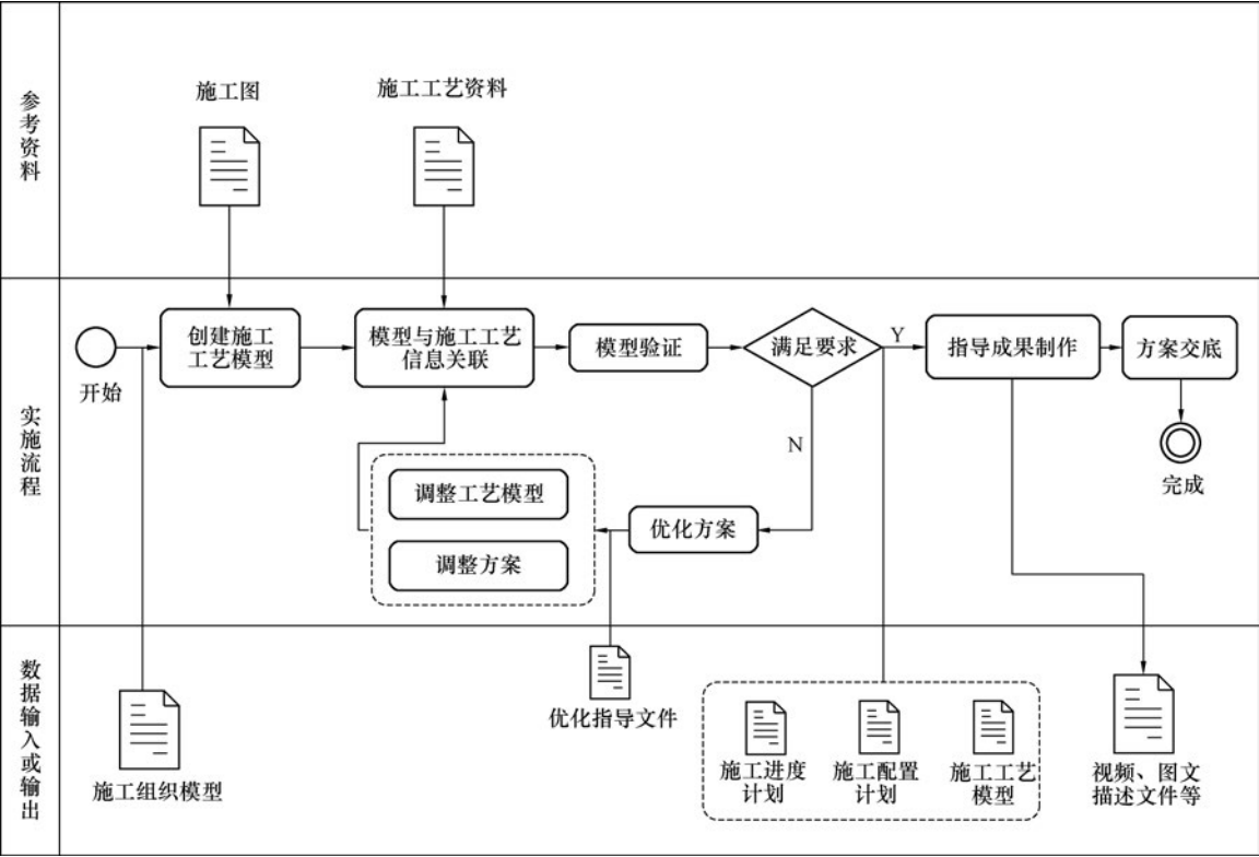
图 7.3.8 施工工艺模拟 BIM 应用流程示意
