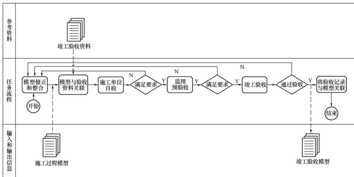
图 12.1.4 竣工验收 BIM 应用流程
