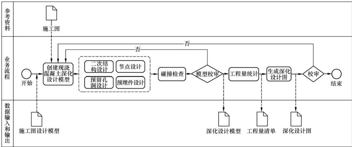
图 6.2.3 现浇混凝土结构深化设计 BIM 典型应用示意
