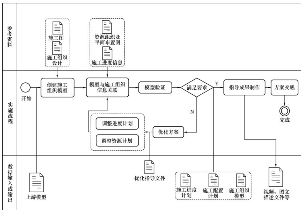
图 7.2.6 施工组织模拟 BIM 应用流程示意
