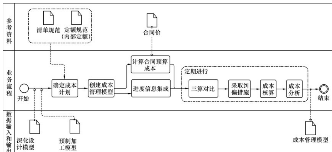
图 9.3.5 成本管理 BIM 应用流程
