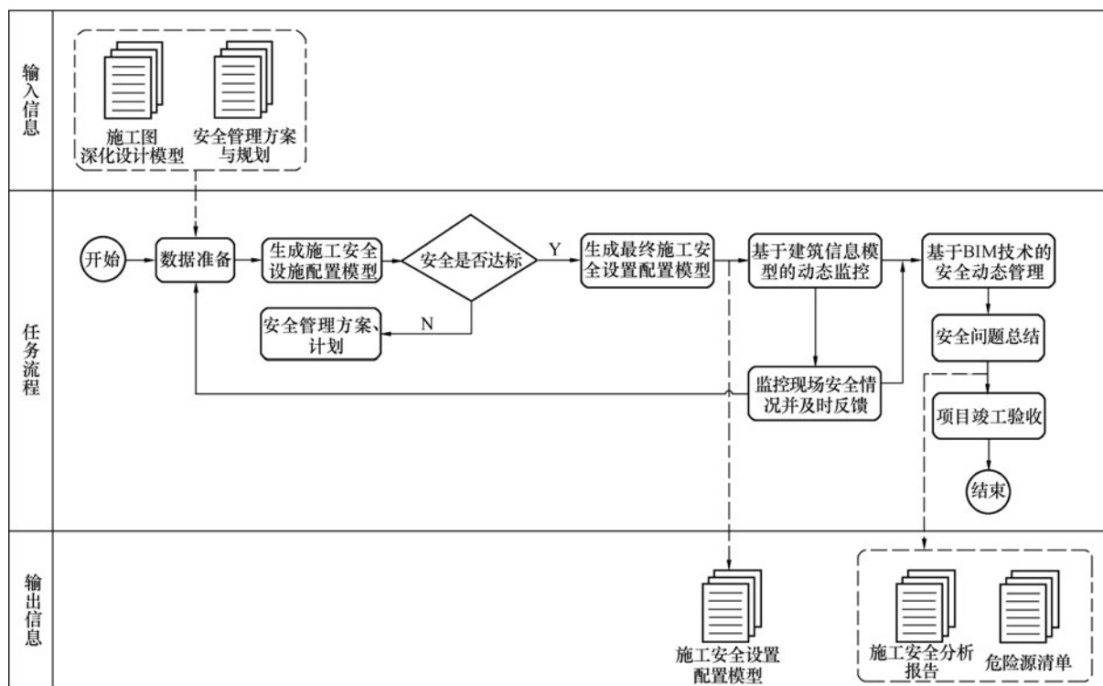
图 10.3.10 安全管理 BIM 应用流程
