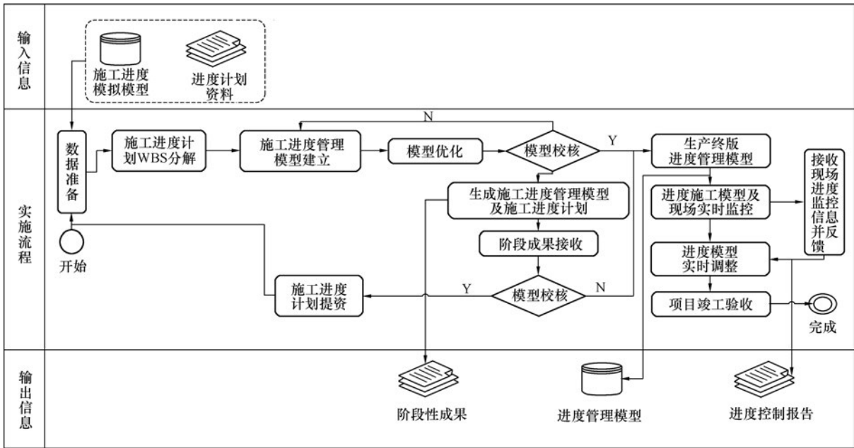
图 8.3.4 施工进度管理 BIM 应用流程
