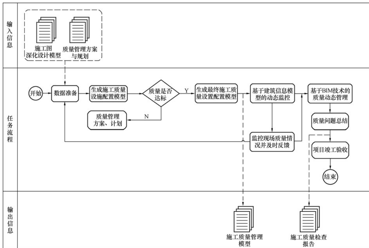
图 10.2.10 质量管理 BIM 应用流程
